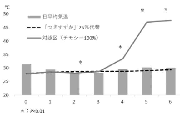
図3 「つきすずか」発酵TMRの開封後6日間の温度
